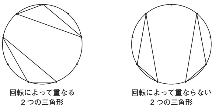
図1. 2つの三角形の関係
