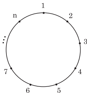
図 3. 円を n 等分する
